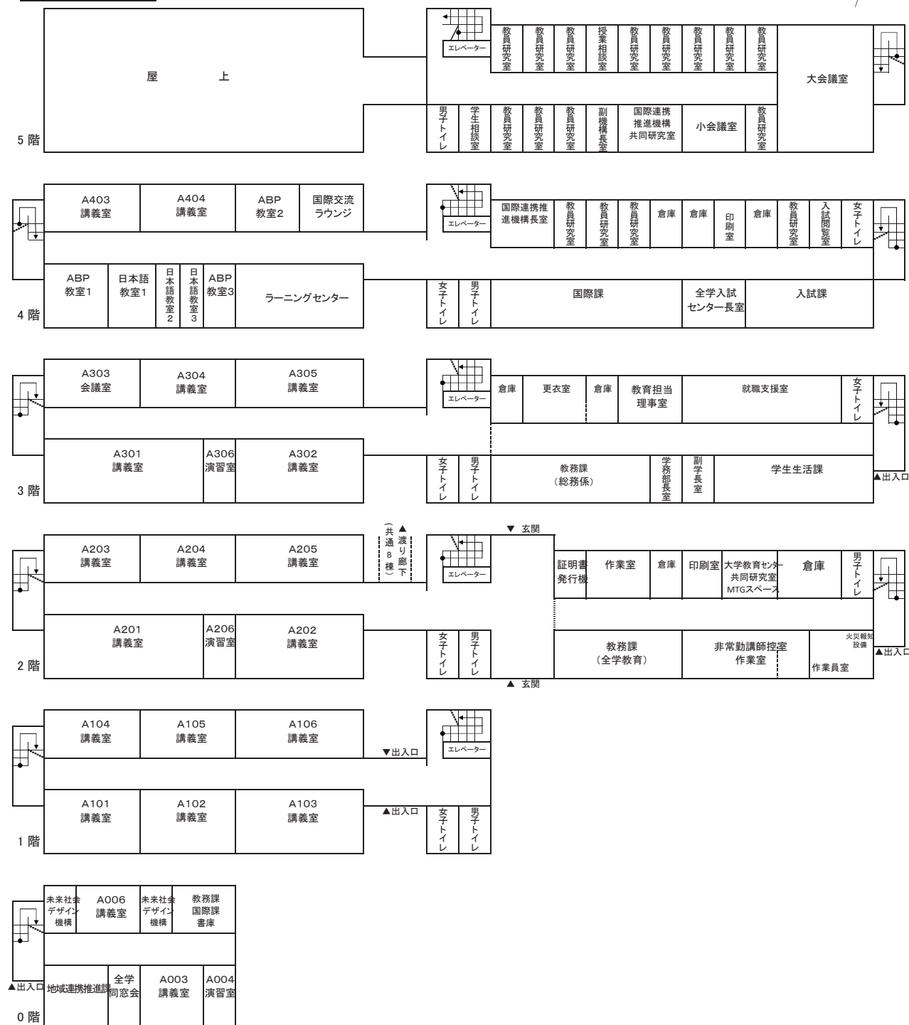
共通教育A棟平面図
